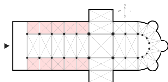
SLIKA 2: Območje stranskih ladij na tlorisu
