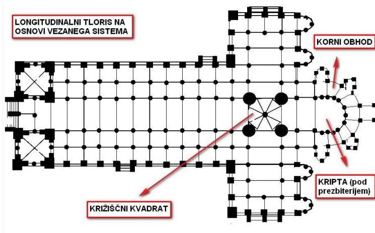
SLIKA 6: Tloris romanske cerkve
